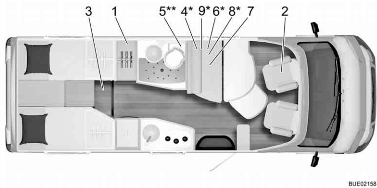
Fig. 295 Tracé Nexxo Time T 690 G
