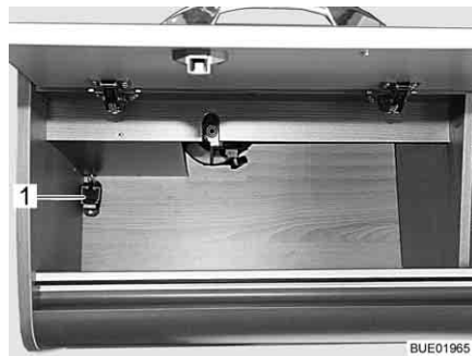
Fig. 179 Fusible du lit escamotable à l'avant
