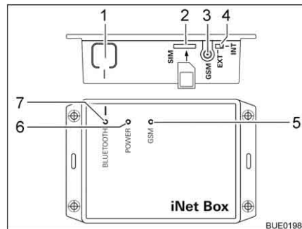
Fig. 212 Truma iNet-Box
