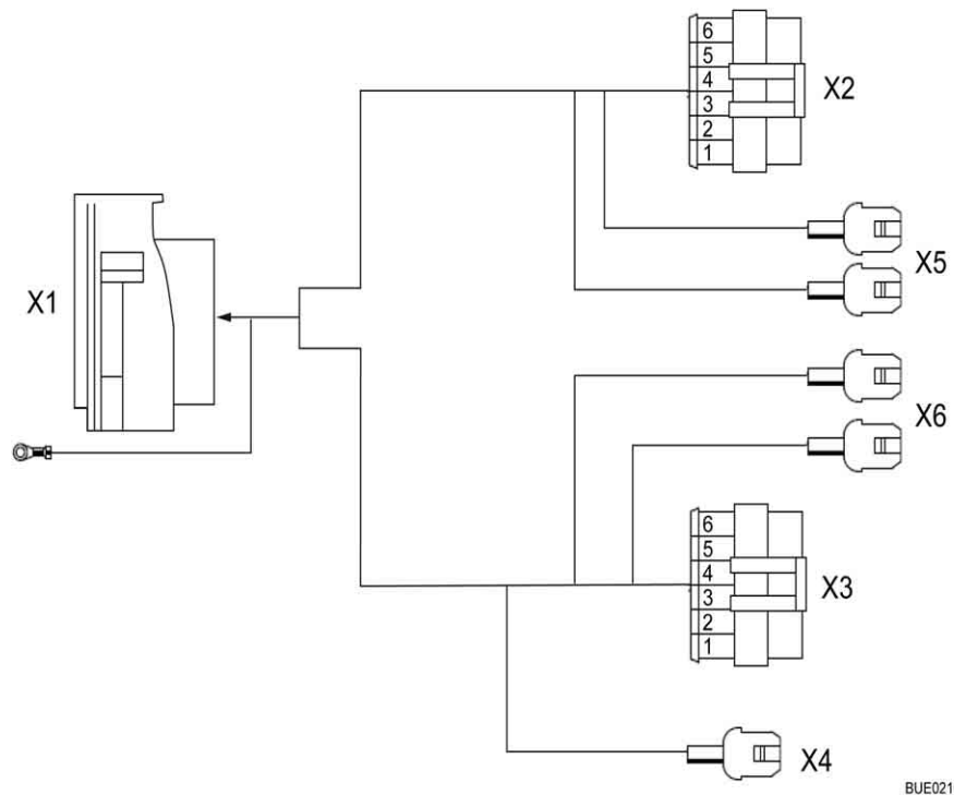
Fig. 187 Schéma électrique extérieur
