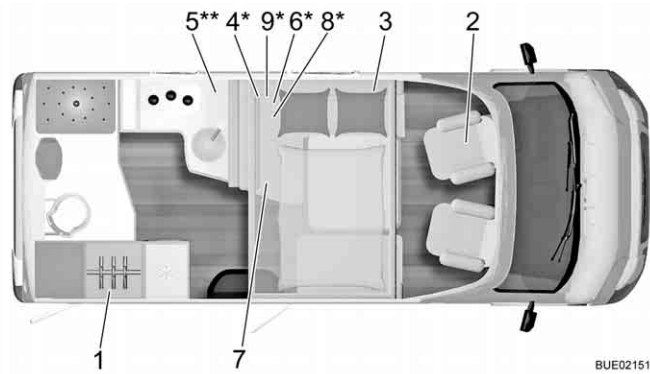
Fig. 296 Tracé Ixeo Time IT 590
