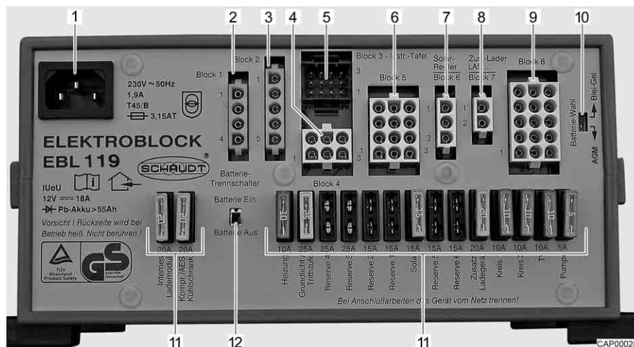
Fig. 166 Bloc électrique (EBL 119)
