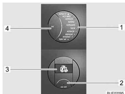
Fig. 36 Panneau de commande (TeleSat)
