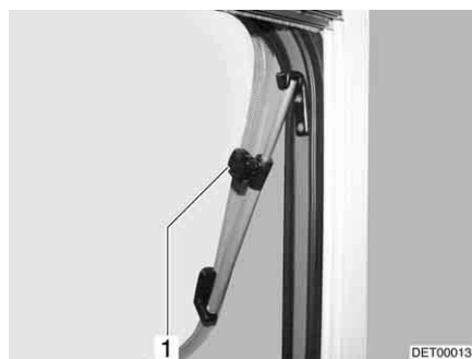
Fig. 81 Fenêtre projetante avec bras pivotant
