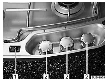
Fig. 214 Boutons de commande pour le réchaud à gaz (alternative)
