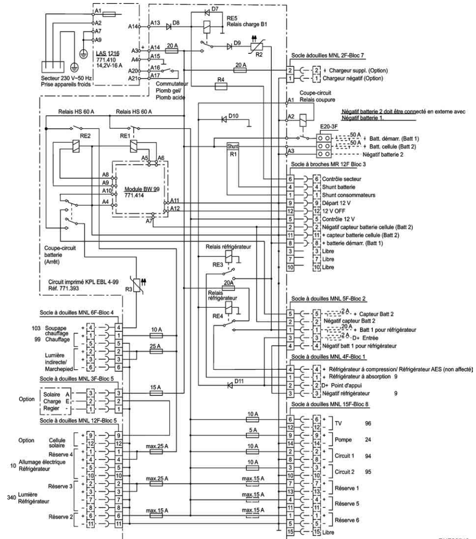
Fig. 122 Schéma électrique intérieur (EBL 99)
