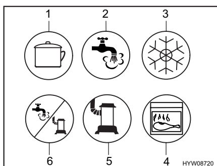
Fig. 96 Symboles possibles des robinets d'arrêt de gaz
