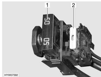
Fig. 112 Fusibles de la batterie de cellule
