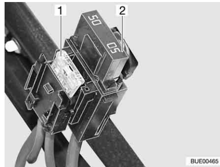
Fig. 111 Fusibles de la batterie de démarrage
