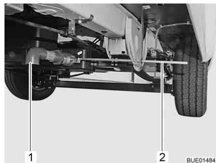
Fig. 160 Robinet de vidange
