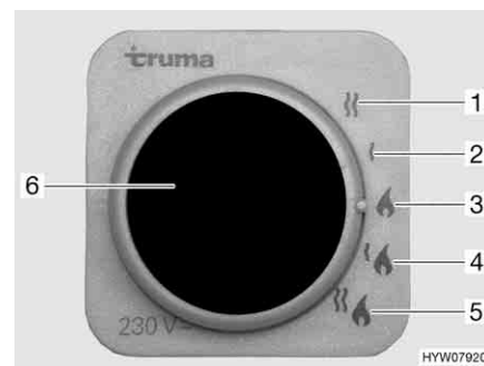
Fig. 142 Sélecteur de source d'énergie pour chauffage/chauffe-eau
