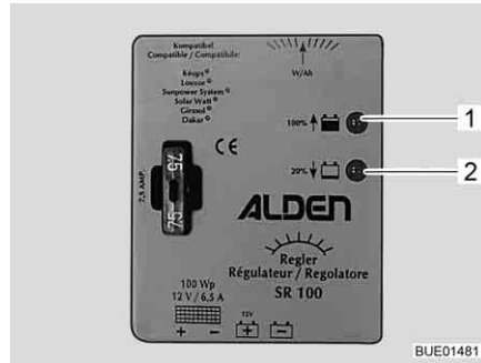
Fig. 106 Régulateur de panneau solaire 100 W
