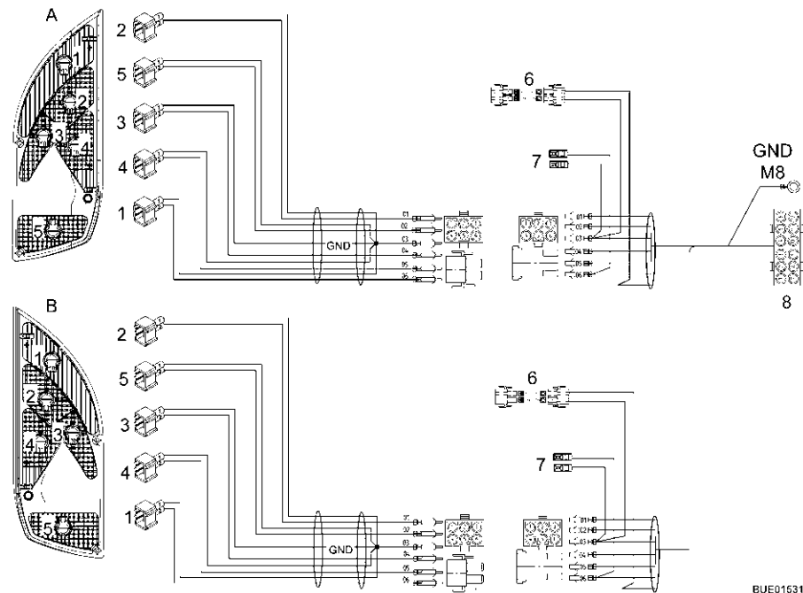
Fig. 124 Schéma électrique extérieur
