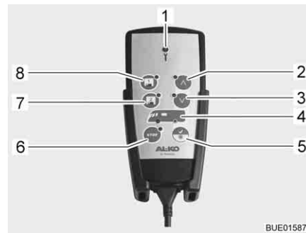
Fig. 25 Télécommande
