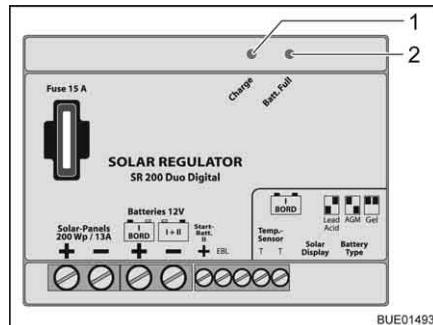
Fig. 141 Régulateur de panneau solaire 200 W
