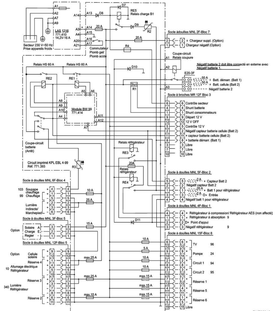
Fig. 157 Schéma électrique intérieur (EBL 99)
