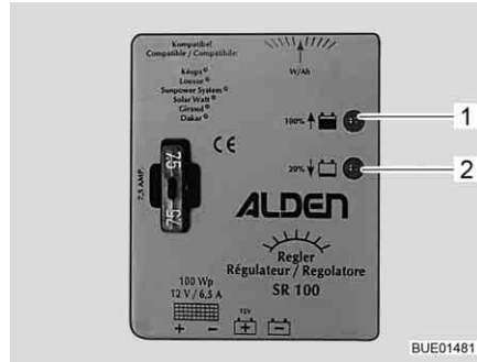
Fig. 140 Régulateur de panneau solaire 100 W
