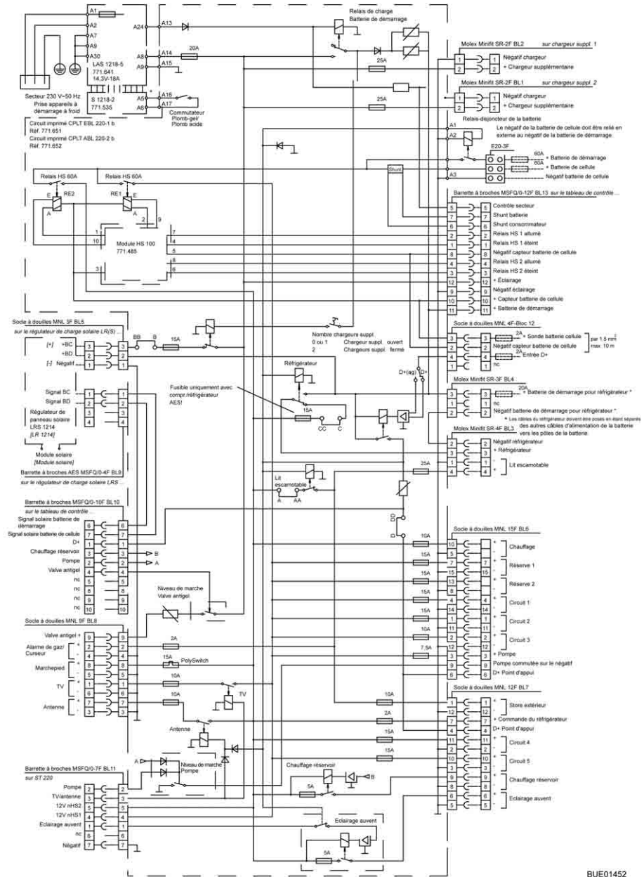
Fig. 158 Schéma électrique intérieur (EBL 220)
