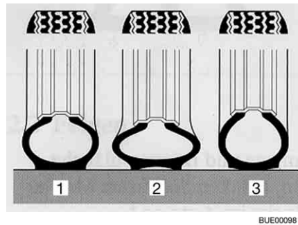
Fig. 251 Surface de contact du pneu
