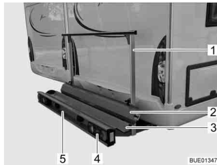
Fig. 8 Porte-charge
