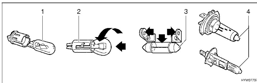
Fig. 230 Types d'ampoules
