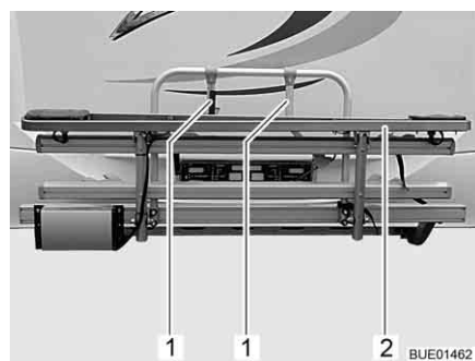
Fig. 5 Porte-vélos e-bike
