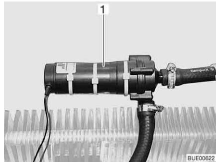
Fig. 171 Circulateur supplémentaire
