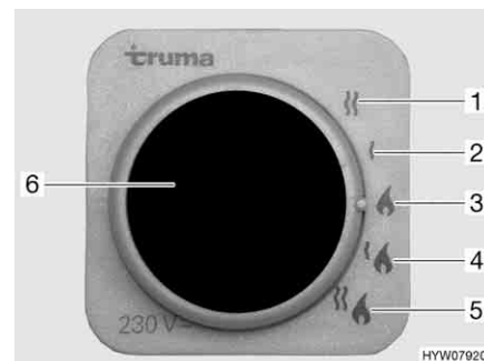
Fig. 140 Selector de energía para la calefacción/caldera
