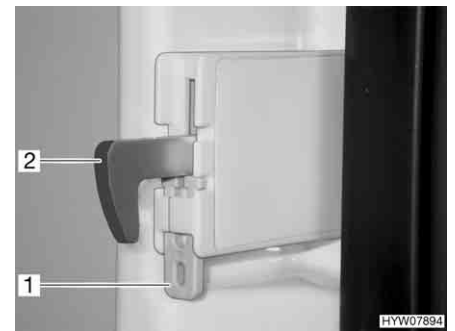
Fig. 146 Fijación del gancho de bloqueo
