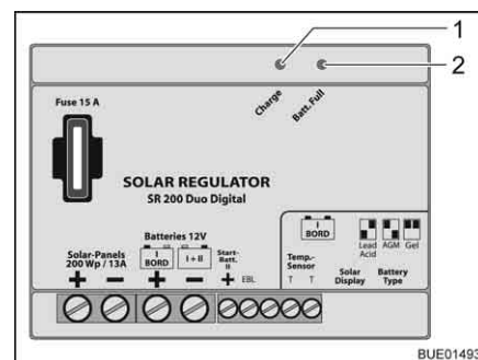
Fig. 108 Regulador de carga solar 200 W
