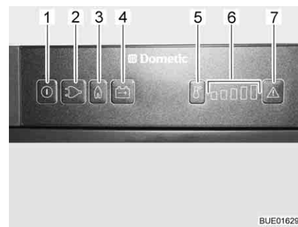
Fig. 144 Elementos de mando para el frigorífico (Dometic de la serie 8 con SMSE)
