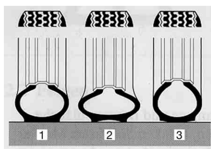
Fig. 187 Superficie de contacto del neumático
