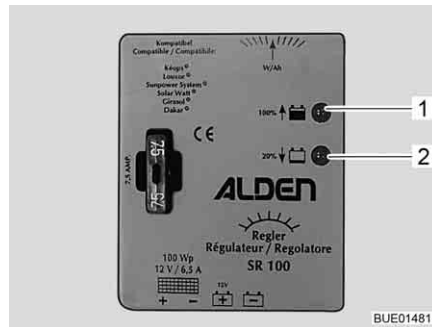
Fig. 107 Regulador de carga solar 100 W
