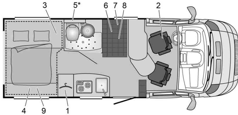
Fig. 188 Esquema T 605 Brevio
