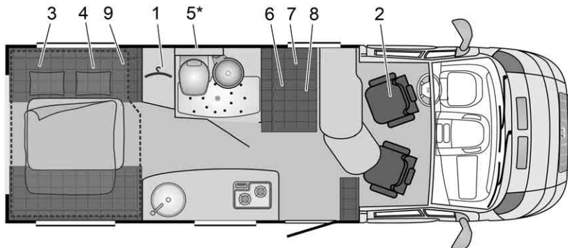
Fig. 190 Esquema T 645 Brevio
