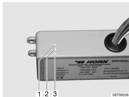
Fig. 154 Aparato regulador
