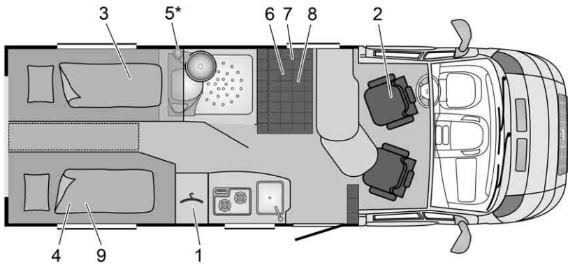
Fig. 189 Esquema T 640 Brevio
