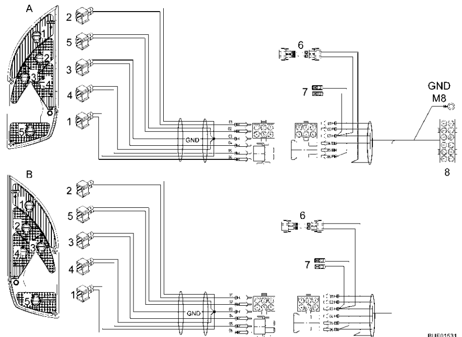
Afb. 125 Stroomschema buiten
