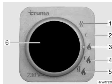
Afb. 140 Energiekeuzeschakelaar voor verwarming/boiler
