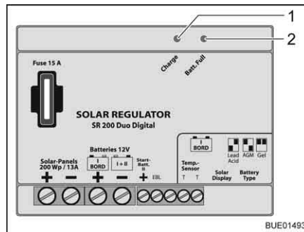
Afb. 108 Zonneregelaar 200 W
