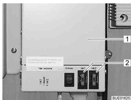
Afb. 116 Regelaar verwarming voor afvalwaterleidingen
