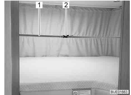
Afb. 88 Hefbed met gesloten spanband
