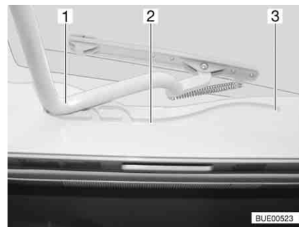
Afb. 68 Heki-dakluik, geleiding
