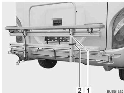
Afb. 1 Fietsenrek (ingeklapt)
