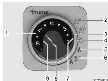
Afb. 128 Bedieningspaneel voor verwarming/boiler
