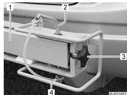
Afb. 2 Vergrendeling fietsenrek
