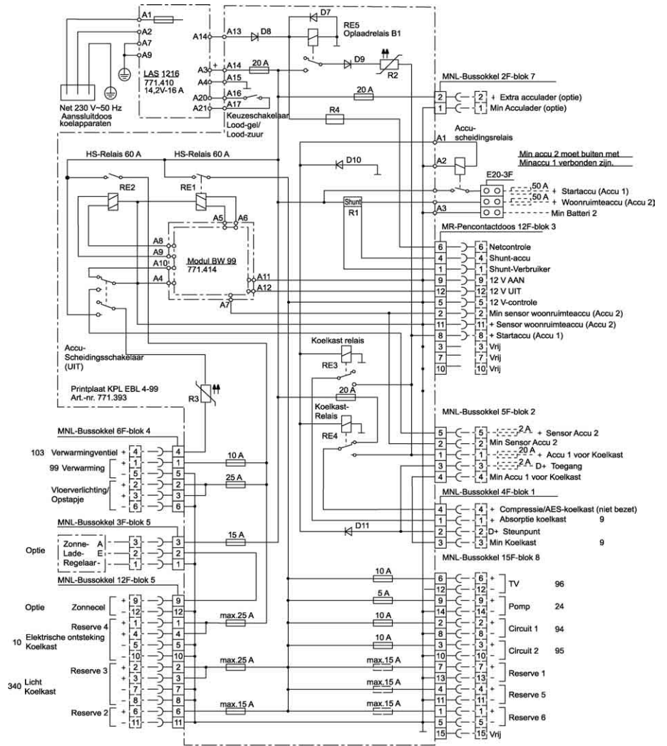
Afb. 123 Stroomschema binnen (EBL 99)
