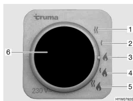
Fig. 194 Sélecteur de source d'énergie pour chauffage/chauffe-eau
