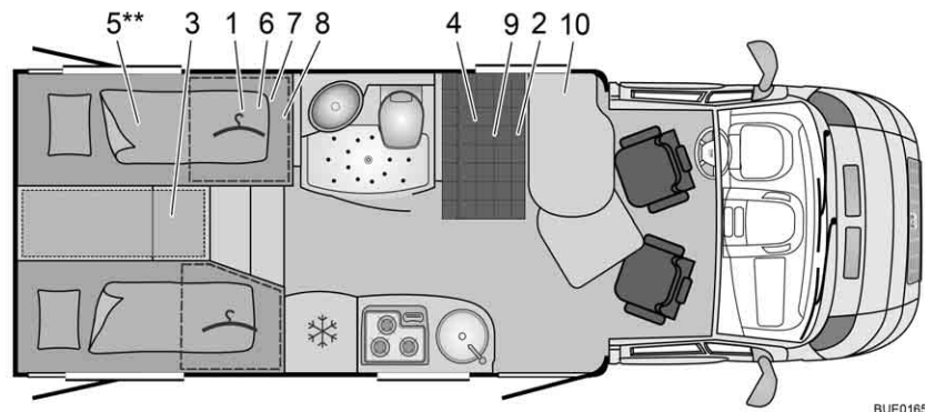
Fig. 294 Tracé T 690 G Nexxo
