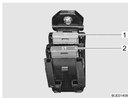
Fig. 181 Fusibles pour pile à combustible
