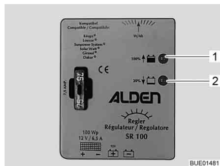
Fig. 171 Régulateur de panneau solaire 100 W
