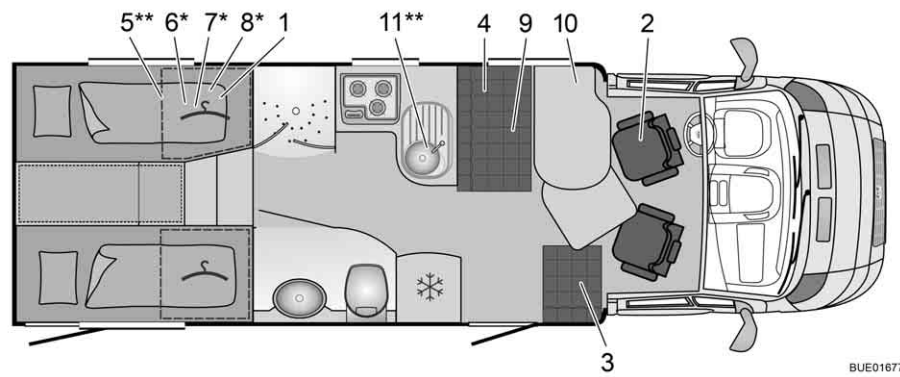
Fig. 300 Tracé T 728 G Nexxo
