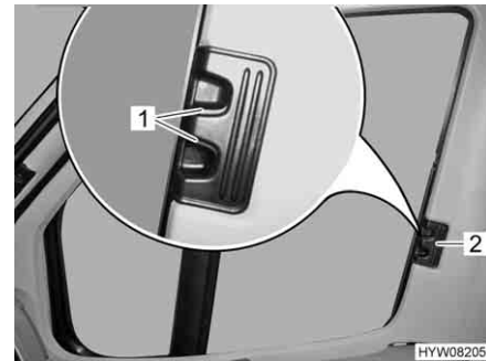
Fig. 35 Dispositif occultant plissé pour la fenêtre côté conducteur/passager
