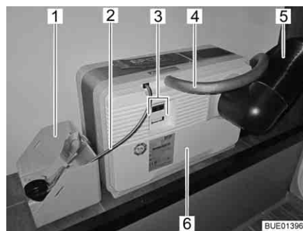
Fig. 168 Pile à combustible avec cartouche de réservoir
