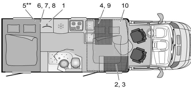
Fig. 297 Tracé IT 710 G Ixeo Time
