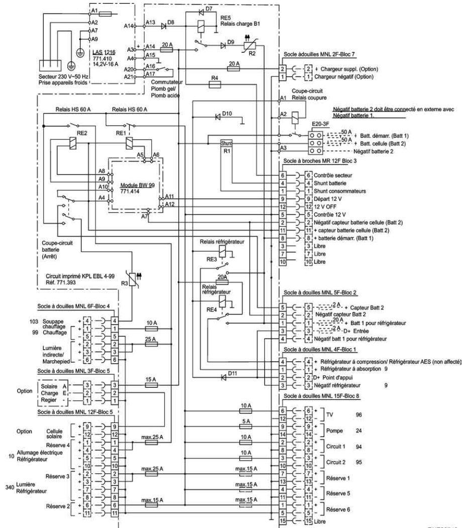
Fig. 188 Schéma électrique intérieur (EBL 99)
