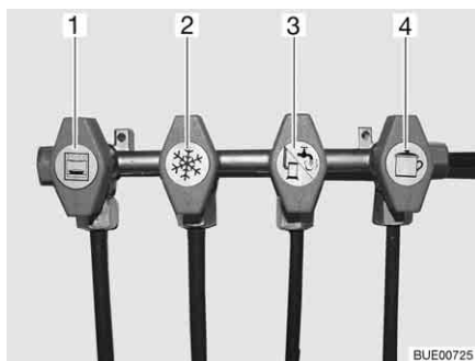
Fig. 158 Symboles des robinets d'arrêt de gaz
