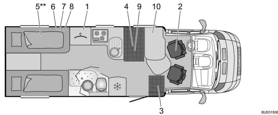
Fig. 301 Tracé T 729 Nexxo
