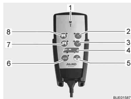
Fig. 27 Télécommande
