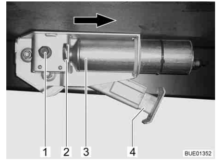
Fig. 40 Vérin stabilisateur électrique sur le véhicule
