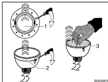
Fig. 270 Remplacer l'ampoule halogène
