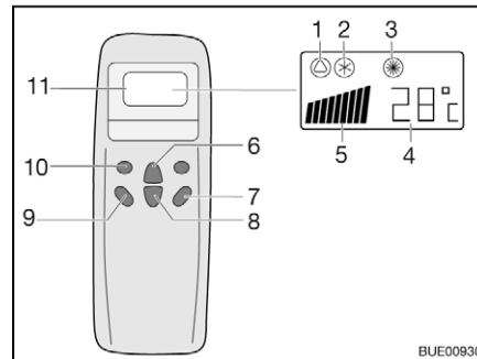
Fig. 210 Télécommande
