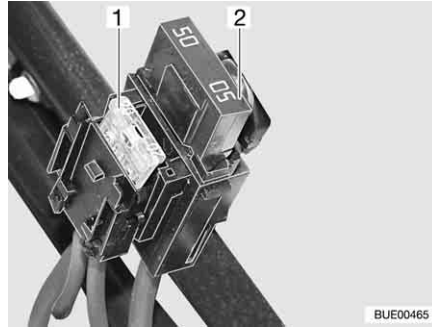
Fig. 176 Fusibles de la batterie de démarrage
