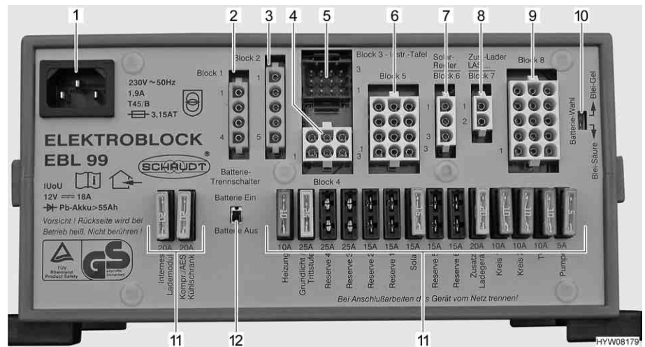
Fig. 166 Bloc électrique (EBL 99)
