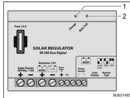
Fig. 172 Régulateur de panneau solaire 200 W
