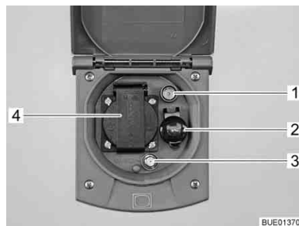
Fig. 185 Prise extérieure
