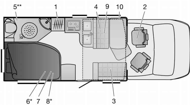
Fig. 292 Tracé IT 664 Ixeo
