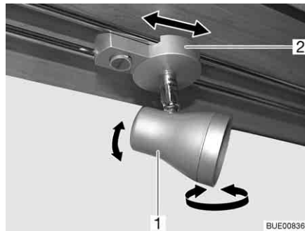
Fig. 58 Faretto
