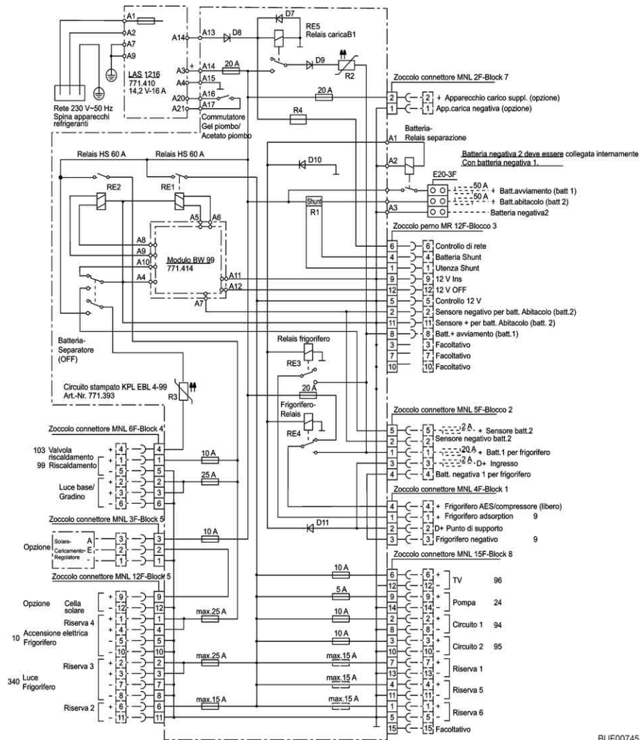
Fig. 135 Schema elettrico interno (EBL 99)
