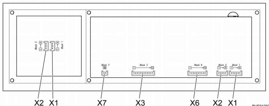
Fig. 138 Schema a blocchi, pannello di controllo (LT 510)
