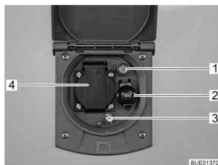
Fig. 132 Presa esterna
