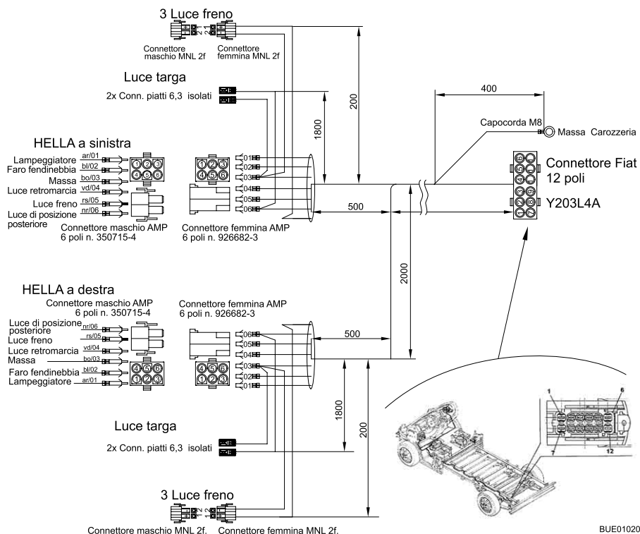
Fig. 139 Schema elettrico esterno
