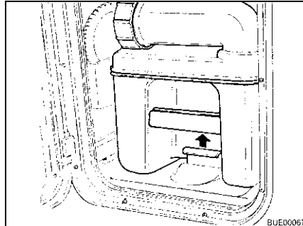
Afb. 205 Bevestigingsbeugel trekken
