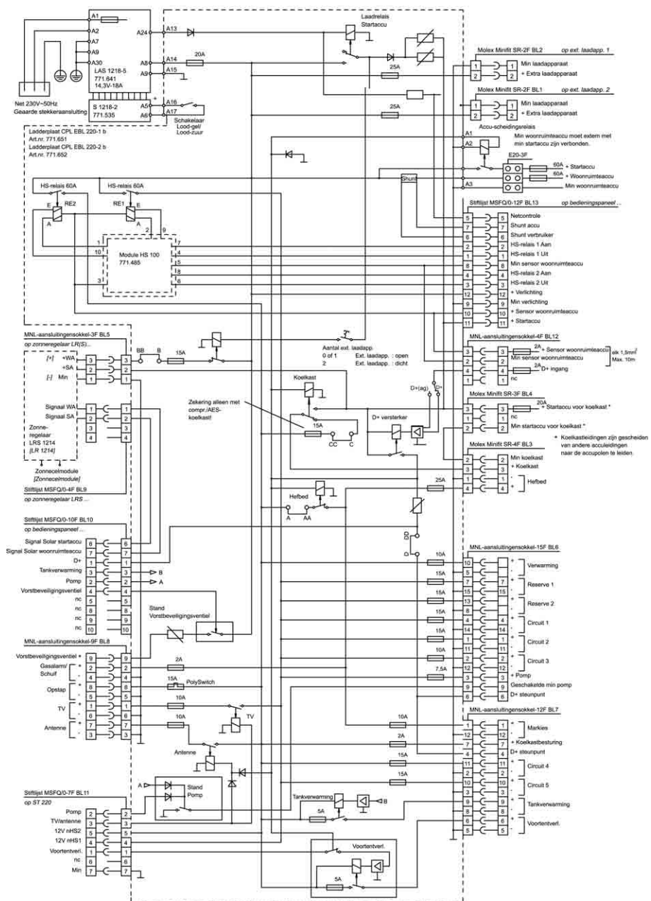
Afb. 136 Stroomschema binnen (EBL 220)
