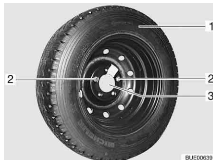
Afb. 240 Reservewielhouder in de garage achter
