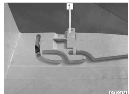
Afb. 80 Vergrendeling ventilatiestand
