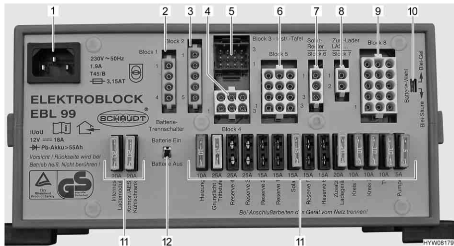
Afb. 115 Elektroblok (EBL 99)
