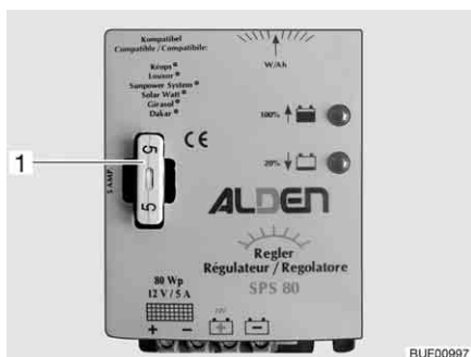
Afb. 130 Zekering zonneregelaar
