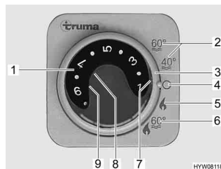
Afb. 142 Bedieningspaneel voor verwarming/boiler
