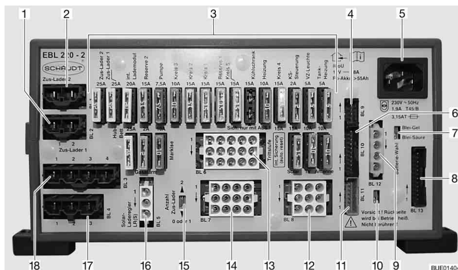
Afb. 116 Elektroblok (EBL 220)
