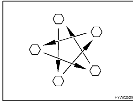
Afb. 234 Wielmoeren of wielschroeven kruisgewijs aandraaien
