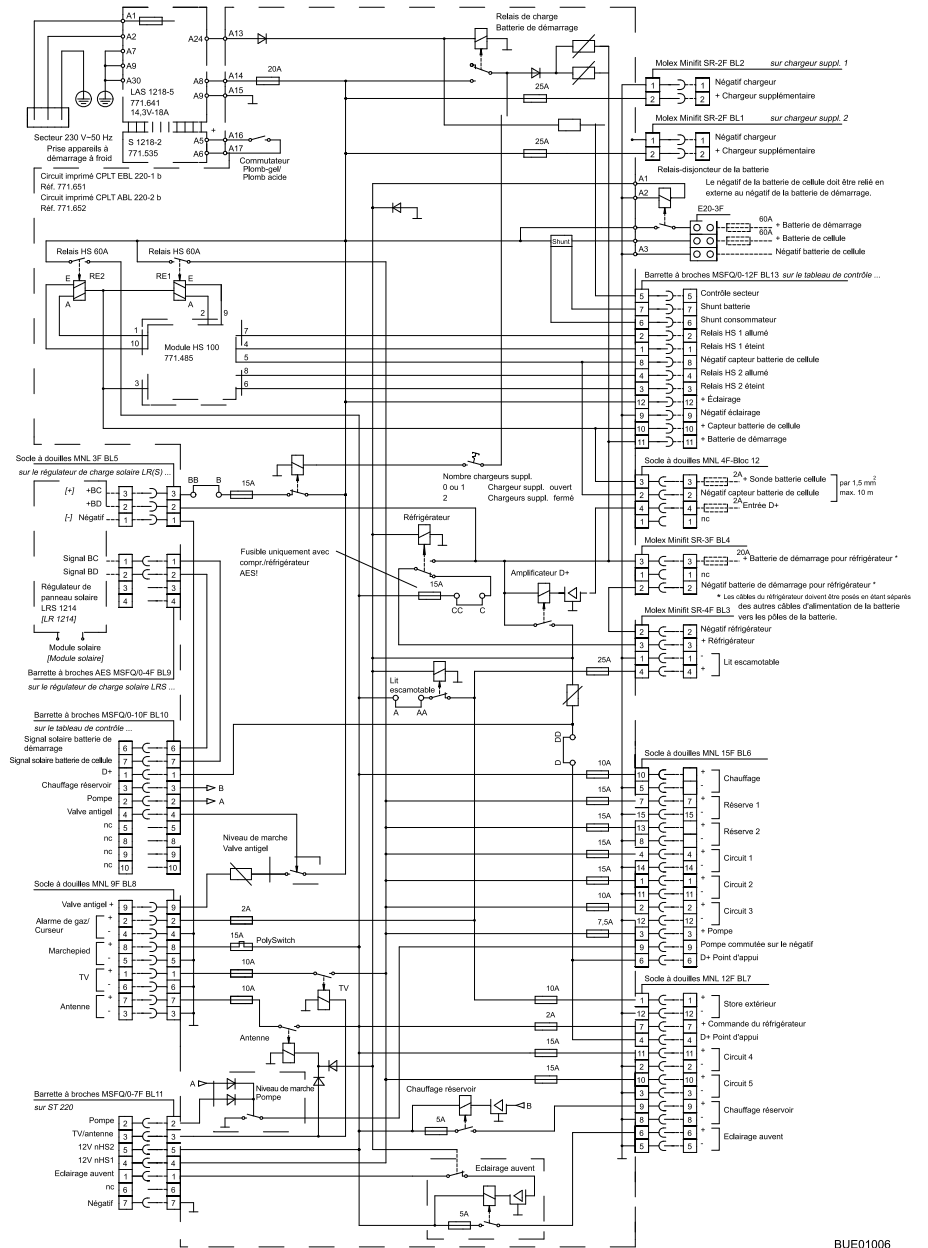
Fig. 122 Schéma électrique intérieur (EBL 220)
