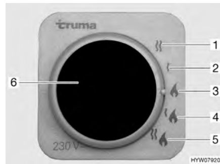
Fig. 147 Sélecteur de source d'énergie pour chauffage/chauffe-eau
