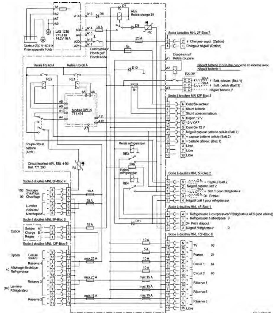
Fig. 121 Schéma électrique intérieur (EBL 99)
