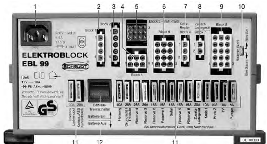
Fig. 102 Bloc électrique (EBL 99)
