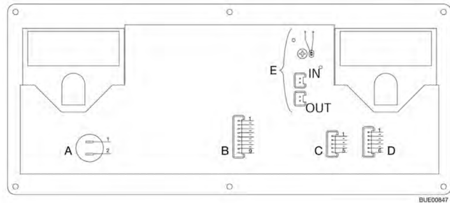
Fig. 123 Schéma fonctionnel panneau de contrôle (IT 994)
