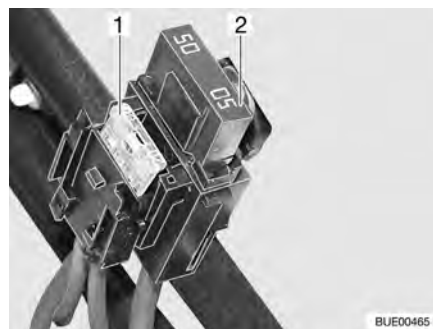
Fig. 112 Fusibles de la batterie de démarrage
