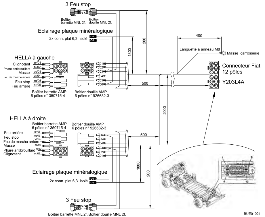
Fig. 126 Schéma électrique extérieur
