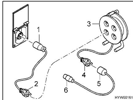
Fig. 109 Possibilités de raccordement 230 V
