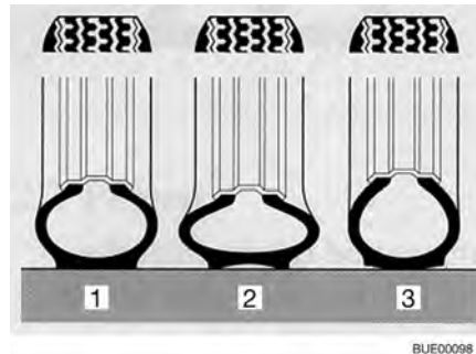
Fig. 214 Surface de contact du pneu
