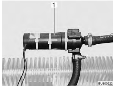
Fig. 135 Circulateur supplémentaire
