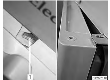
Fig. 161 Porte du réfrigérateur/du compartiment congélation en position de ventilation (Dometic Série 7 avec compartiment congélation séparé)
