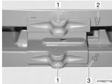
Fig. 160 Verrouillage de la porte du réfrigérateur/du compartiment congélation (Dometic Série 7 avec compartiment congélation séparé)
