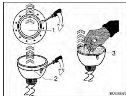
Fig. 203 Remplacer l'ampoule halogène
