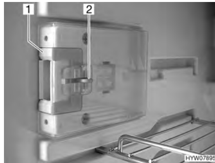
Fig. 164 Dispositif de fermeture en position normale
