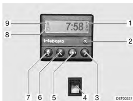
Fig. 140 Unité de commande pour le chauffage d'appoint
