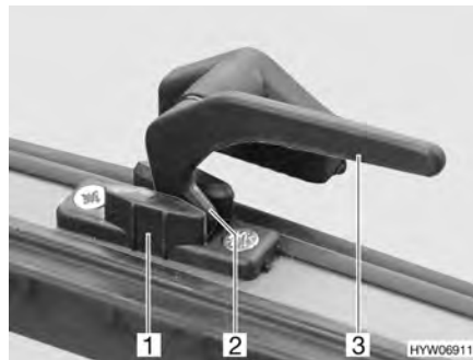
Fig. 56 Palanca de bloqueo en la posición de "ventilación continua"
