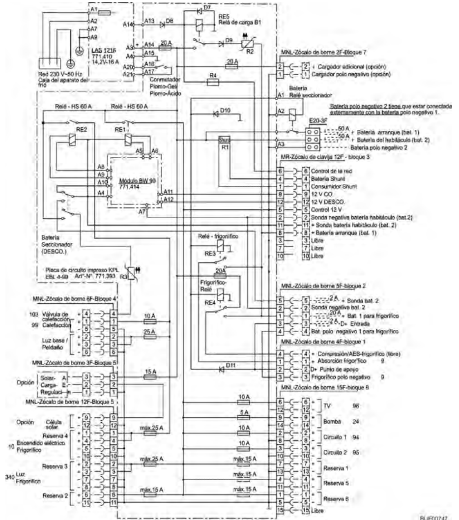
Fig. 121 Esquema de circuitos interior (EBL 99)
