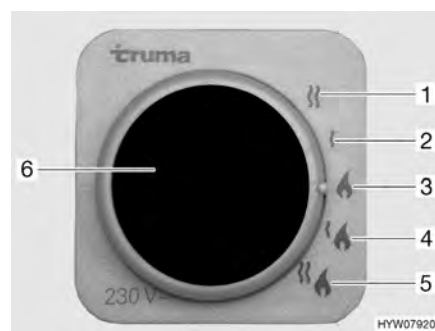
Fig. 130 Selector de energía para la calefacción/caldera
