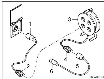
Fig. 109 Posibilidades de conexión de 230 V
