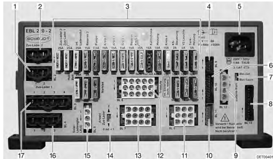
Fig. 103 Bloque eléctrico (EBL 220)
