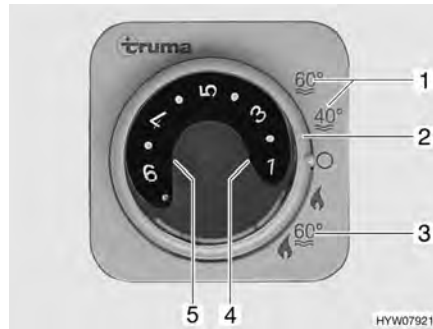
Fig. 145 Unidad de mando para la calefacción/caldera
