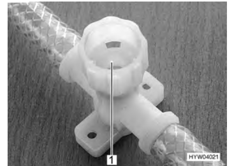
Fig. 172 Llave de desagüe (con tapa giratoria)
