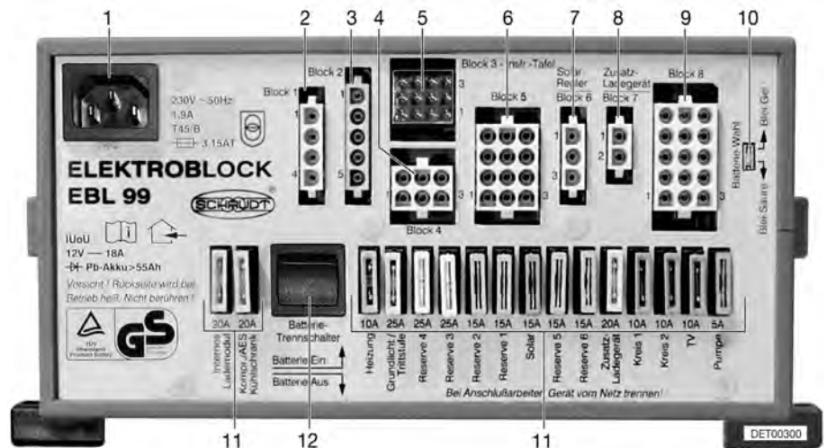
Fig. 102 Bloque eléctrico (EBL 99)
