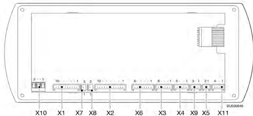
Fig. 124 Diagrama de bloques del panel (DT 220)
