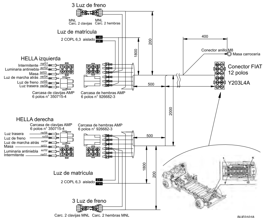
Fig. 126 Esquema de circuitos exterior
