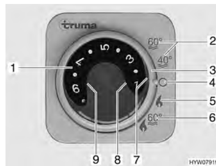
Fig. 129 Unidad de mando para la calefacción/caldera
