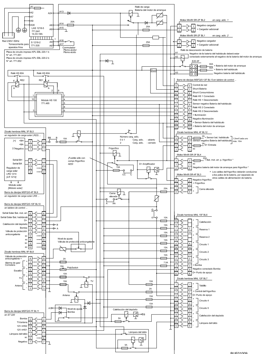
Fig. 122 Esquema de circuitos interior (EBL 220)
