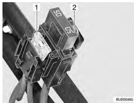
Fig. 112 Fusibles en la batería del motor de arranque
