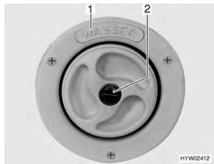
Fig. 34 Tapa de cierre para el tubo de llenado de agua potable
