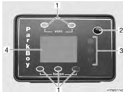
Fig. 15 Unidad de mando del control de distancia de aparcamiento
