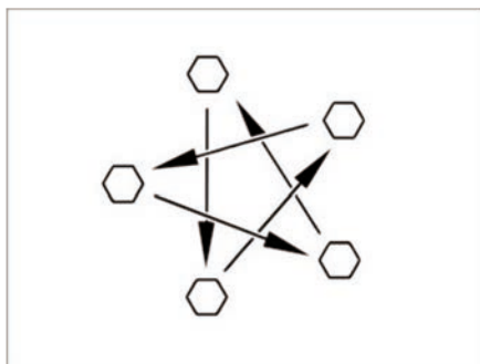
Fig. 156: Apretar mediante cruz las tuercas de rueda o los tornillos de rueda
