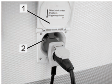
Fig. 95: Conexión de red
