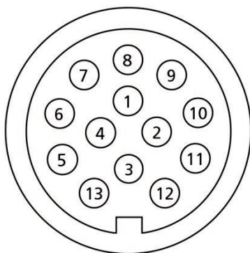
Fig. 2: Conector de 13 polos
