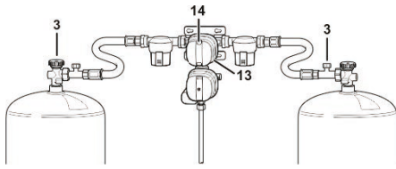
Fig. 106: Juego de regulador de presión de gas
