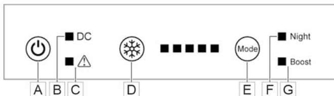
Fig. 155: Elementos de mando de la nevera con compresor de 12 V
