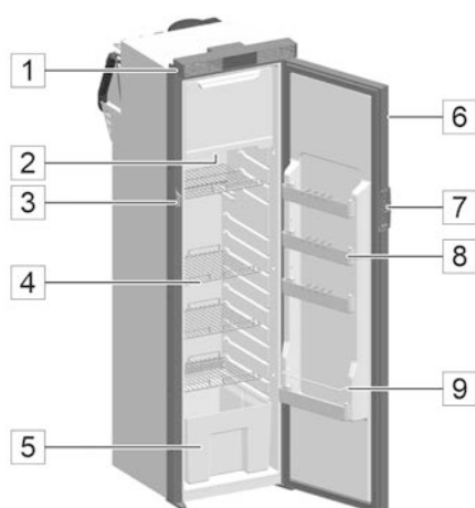
Fig. 154: Nevera con compresor de 12 V
