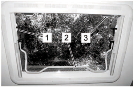
Fig. 121: Manejar el techo para elevar y girar Heki 2
