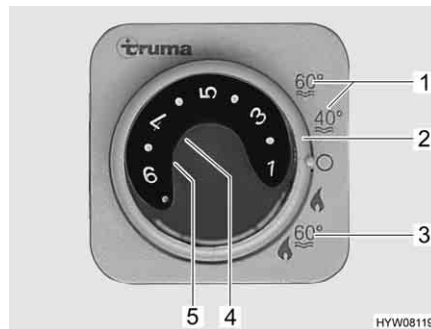
Fig. 176 Unité de commande pour chauffage/chauffe-eau
