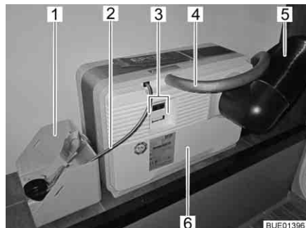
Fig. 134 Pile à combustible avec cartouche de réservoir
