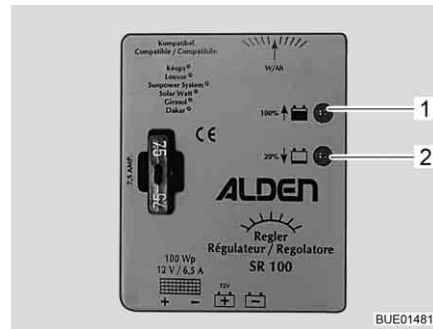
Fig. 137 Régulateur de panneau solaire 100 W
