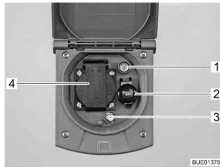
Fig. 149 Prise extérieure
