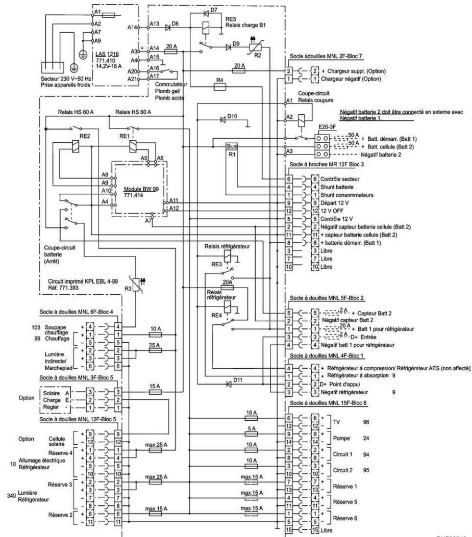
Fig. 152 Schéma électrique intérieur (EBL 99)
