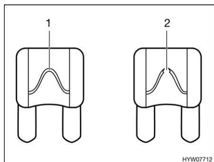
Fig. 141 Fusible 12 V
