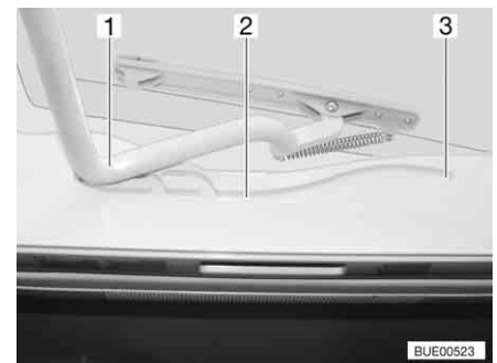
Fig. 90 Lanterneau Heki, glissière
