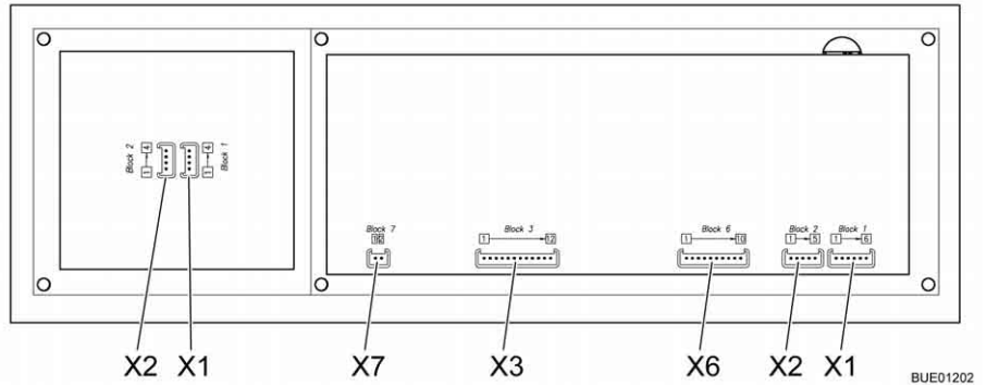
Fig. 155 Schéma fonctionnel, panneau de contrôle (LT 510)
