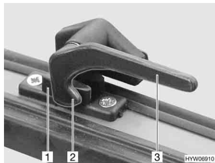
Fig. 96 Levier de verrouillage en position "Fermé"
