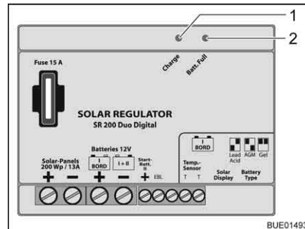
Fig. 138 Régulateur de panneau solaire 200 W
