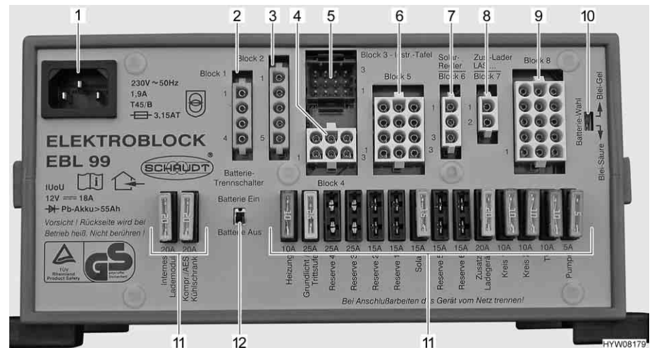
Fig. 130 Bloc électrique (EBL 99)
