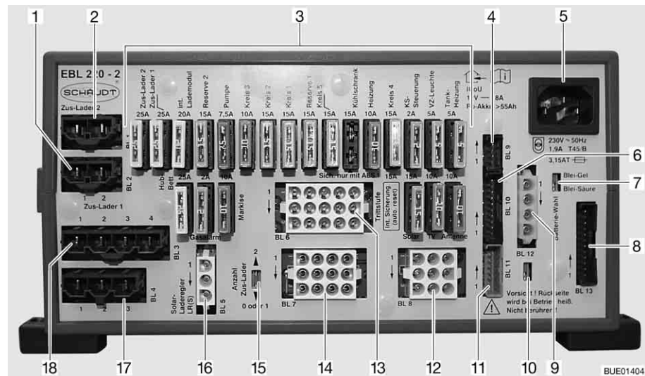
Fig. 131 Bloc électrique (EBL 220)
