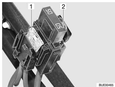
Fig. 142 Fusibles de la batterie de démarrage
