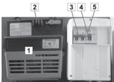
Fig. 58: Convertitore (alimentatore di rete) (1) e interruttori automatici
