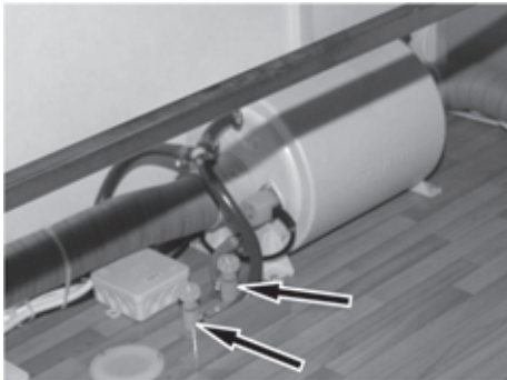
Fig. 121: Valvole di scarico
