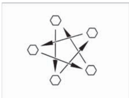
Fig. 146: Serrare in sequenza incrociata i dadi o i bulloni di fissaggio ruota
