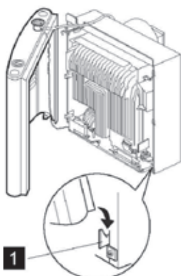
Fig. 116: Rivestimento del riscaldamento aperto
