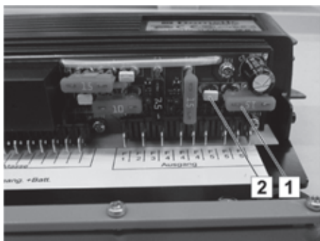
Fig. 59: Illuminazione di emergenza 12 V
