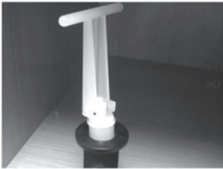
Fig. 92: Tappo di scarico nel serbatoio dell'acqua fresca, aperto (bilanciere diritto)
