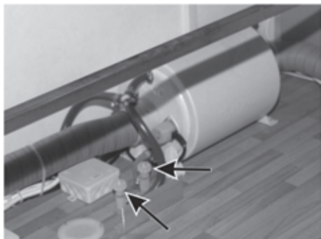
Fig. 86: Boiler TRUMA e valvole per il deflusso dell'acqua
