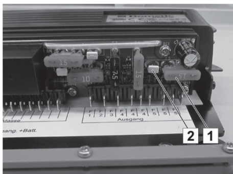
Abb. 56: 12 V-Notbeleuchtung
