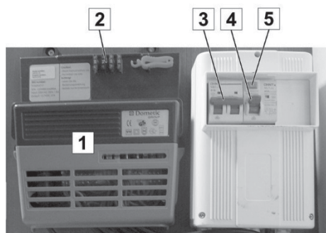
Abb. 55: Umformer (Netzgerät) (1) und Sicherungsautomaten
