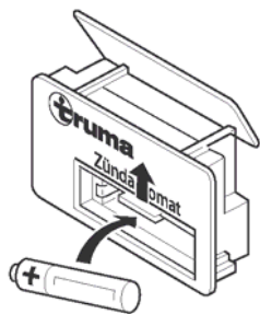
Abb. 109: Batteriewechsel
