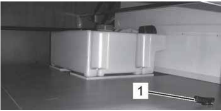
Abb. 89: Ablasshahn (1)
