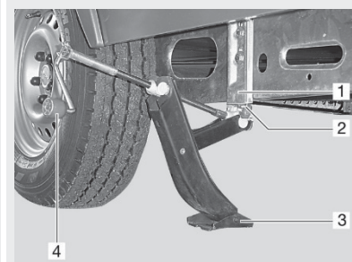
Abb. 142: Wagenheber AL-KO
