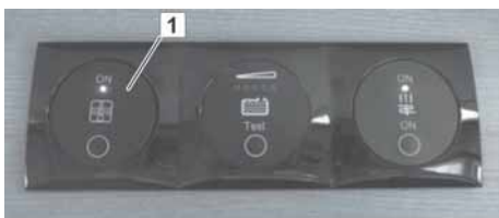
Abb. 114: Ein-/Aus-Schalter der Warmwasserbereitung
