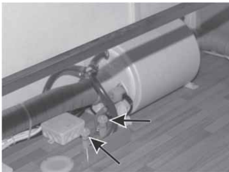
Abb. 82: TRUMA-Therme und Wasserablassventile
