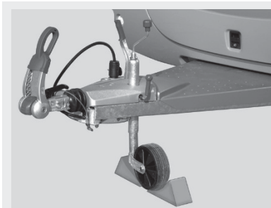
Abb. 139: Stützrad sichern
