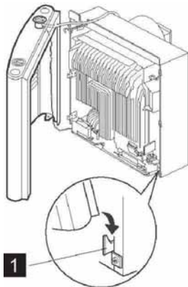
Fig. 108: Open heater grille
