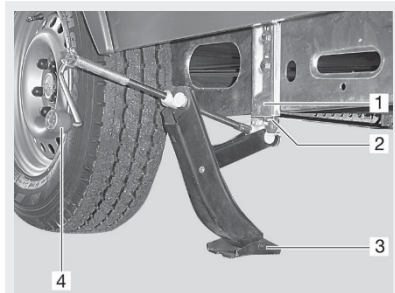
Fig. 142: AL-KO lift jack
